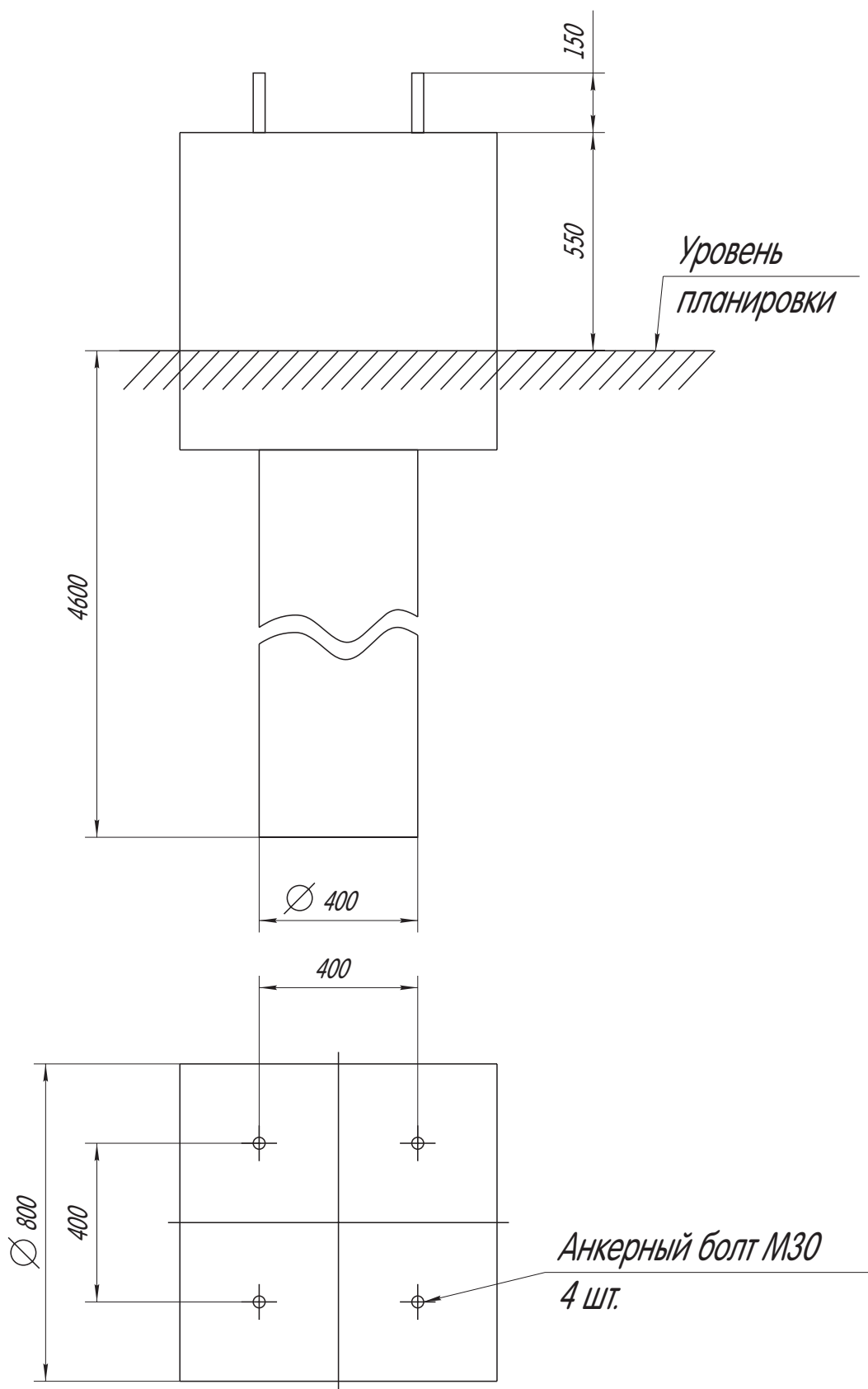
Рисунок 3. Бурунабивной фундамент СФ1.
