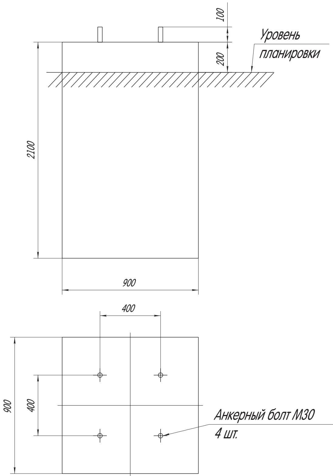
Рисунок 2. Заглубленный фундамент ФМ1-1.
