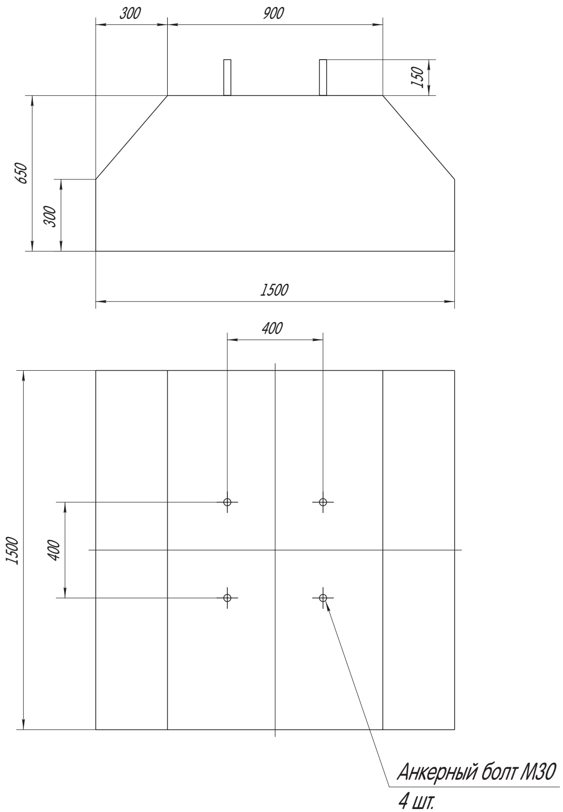
Рисунок 1. Опора ОП1-1.
